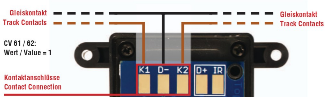
Abbildung 11: Verwendung der Kontaktanschlüsse als Eingang mit Gleiskontakten Figure 11: Using the Auxilliary Contacts as Inputs with Track Contacts
