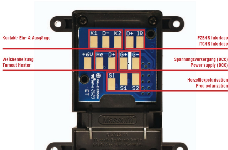
Abbildung 8: Anschlussplatine EVO-X Figure 8: Connection Board EVO-X
