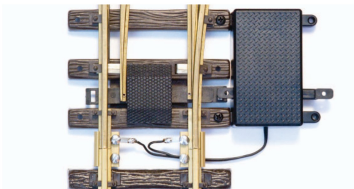
Abbildung 6: Anschluss des Weichenantriebs am Digitalgleis Figure 6: Connecting the Switch Drive to the digital track
