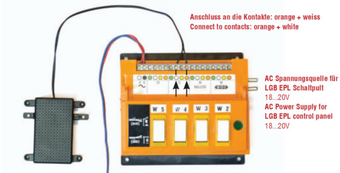
Abbildung 7: Beispielhafter Anschluss des EVO-S an einem EPL Schaltpult Figure 7: Exemplary connection of the EVO-S to an EPL control panel
