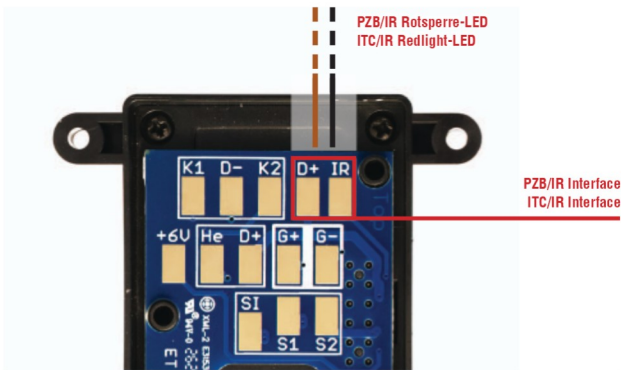
Abbildung 10: Anschluss PZB/IR Rotsperre LED als PZB/IR Signaldecoder Figure 10: Connection the ITC/IR Redlight LED als ITC/IR Signaldecoder
