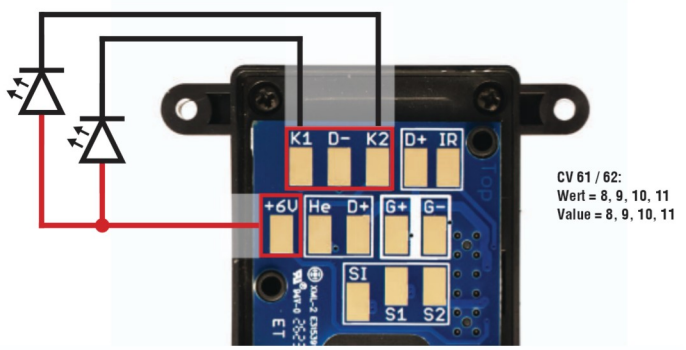
Abbildung 13: Anschluss von LEDs zum Anzeigen der Schaltrichtung (+ geschaltet) Figure 13: Connection of LEDs to indicate the switching direction (+ switched)
